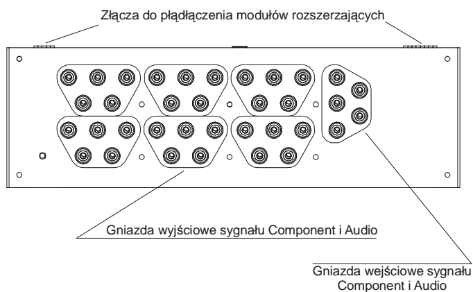
Rys.1 Widok modułu master z góry
